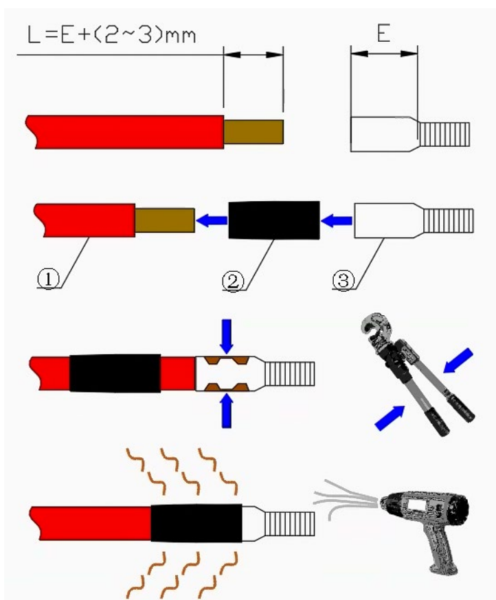
图 6-4 储能机柜PV线压接 ①：线束 ②：热缩管 ③：端子
