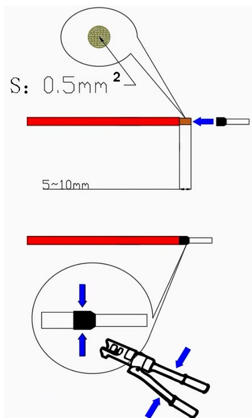
图 6-6 储能机柜通讯线压接（KYT25kW-60kWh-A为例）
