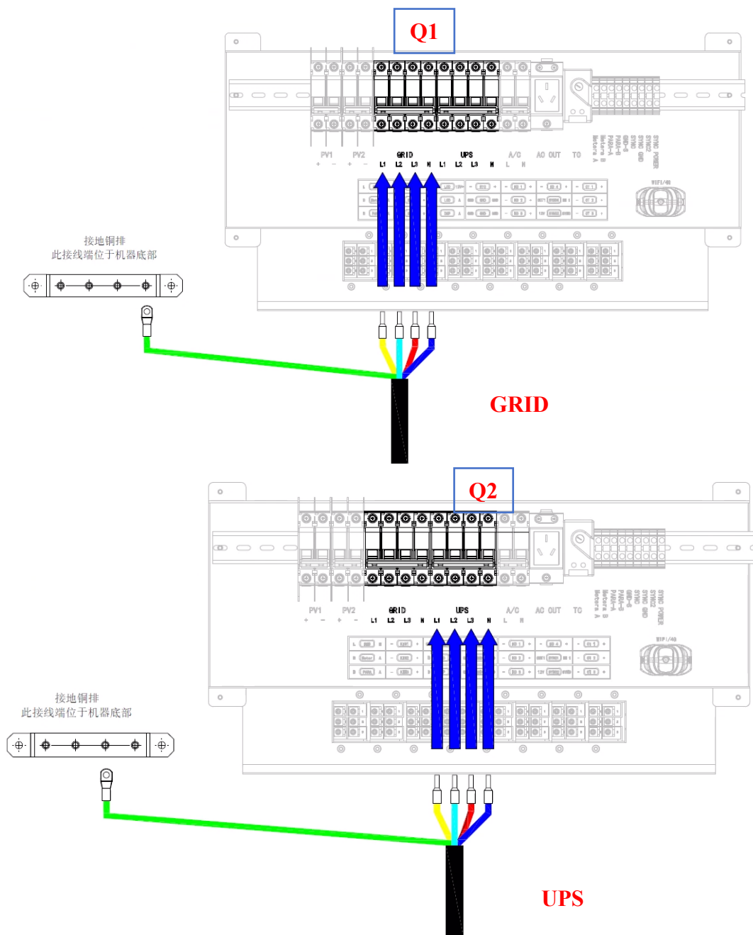
图 6-3 储能机柜AC接线位置（KYT25kW-60kWh-A为例）
