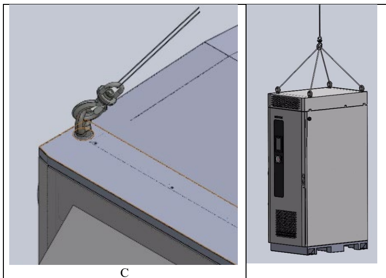
图 5-2 储能机柜吊顶示意
