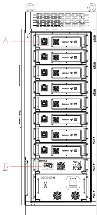
图 7-1 储能机柜操作开关位置总览
