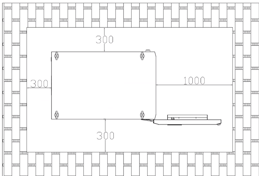
图 5-8 储能机柜周围无遮挡范围尺寸(单位:mm)
