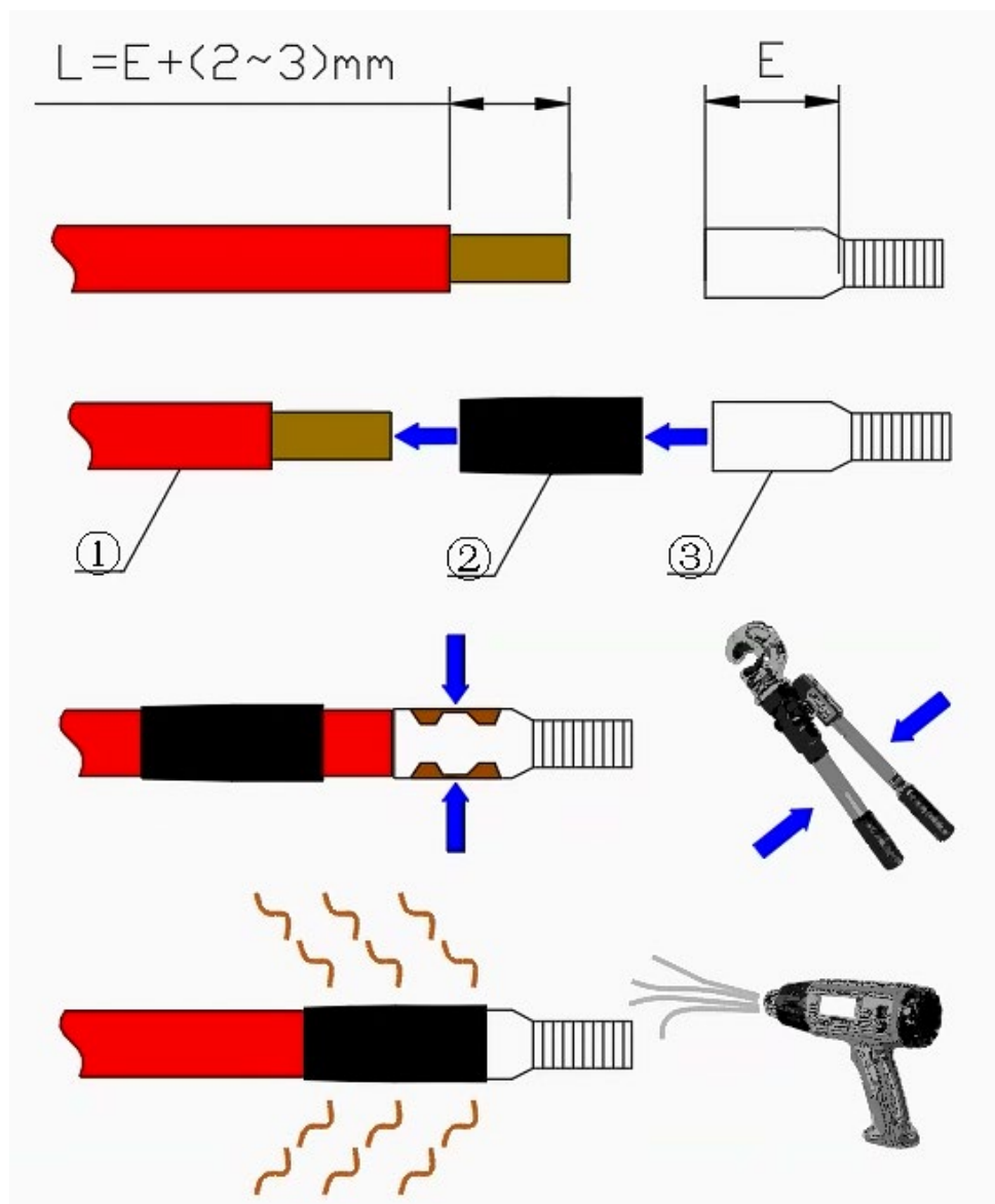
图 6-2 储能机柜交流线压接 ①：线束 ②：热缩管 ③：端子（KYT25kW-60kWh-A为例）
