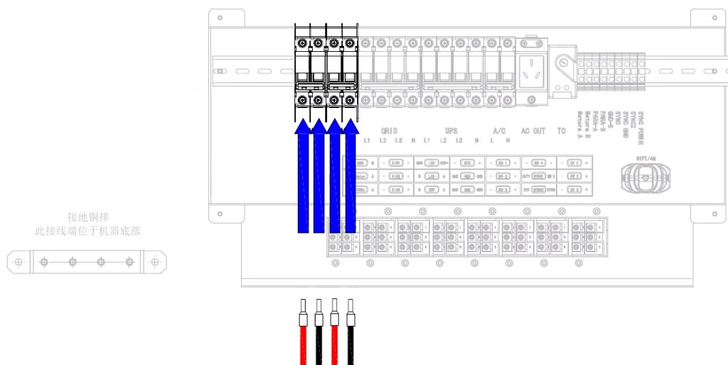
图 6-5 储能机柜PV接线位置（KYT25kW-60kWh-A为例）
