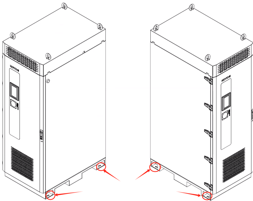
图 5-7 储能机柜固定位置
