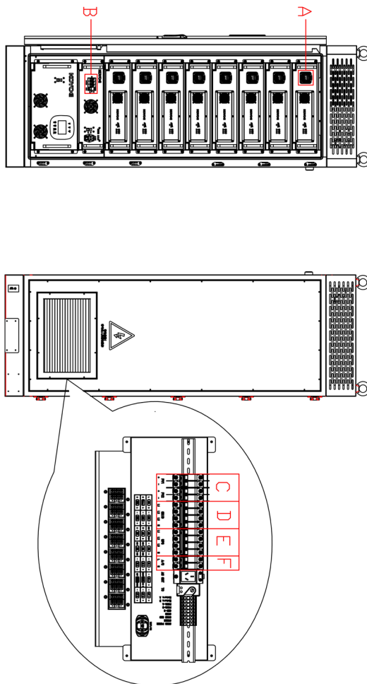
图 3-5 操作开关位置总览（KYT25kW-60kWh-A为例）
