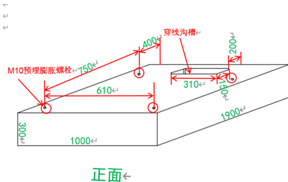
图 5-5 储能机柜设备水泥基础形式1尺寸图 单位：mm
