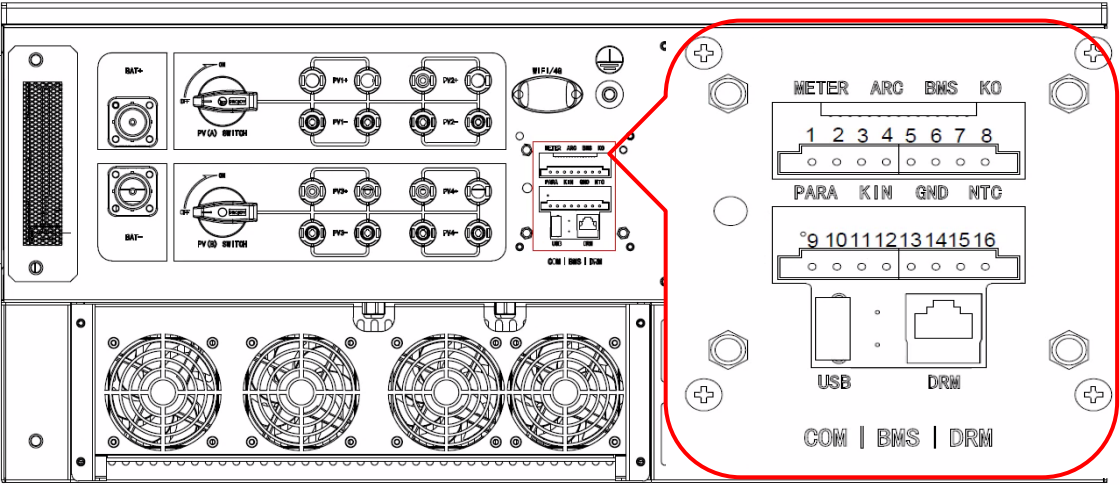
图 6-7 储能机柜通讯接线位置（KYT30kW-108kWh-A为例）
