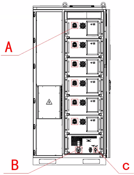
A. MSD； B. 电池开关； C. 电源开关；
