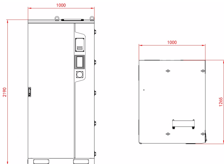
图 3-3 储能机柜尺寸（KYT30KW-108kWh-A为例）
