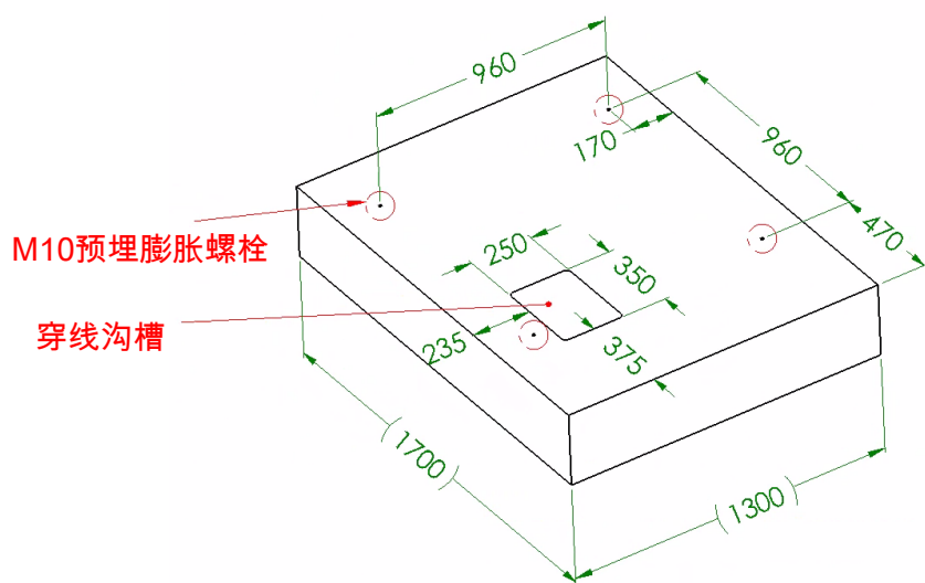
图 5-6 储能机柜设备水泥基础形式2尺寸图（单位：mm）
