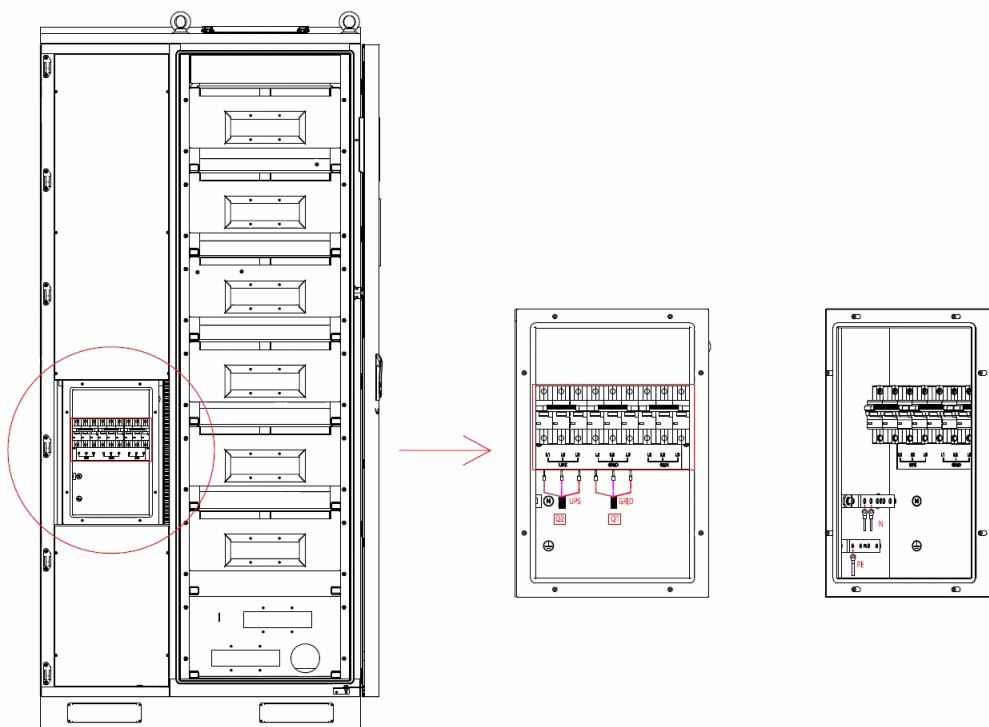
图 6-3 储能机柜AC接线位置
