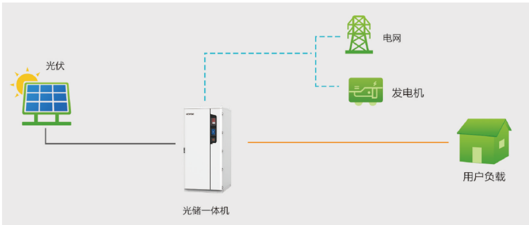
图 3-1 系统示意图
