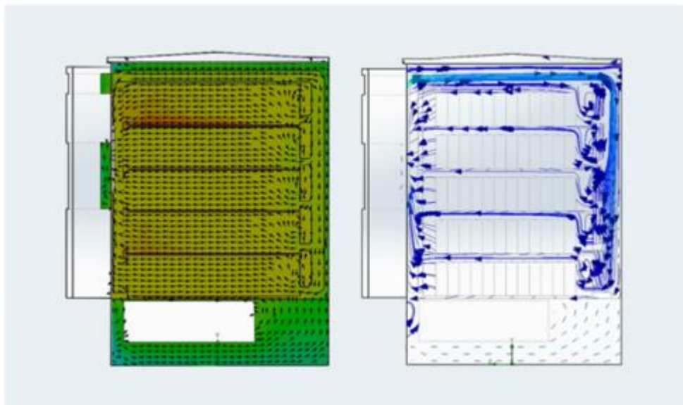
图 3-5 储能机柜热量运行图（KYT30KW-108kWh-A为例）
