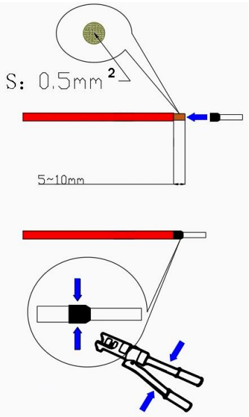
图 6-6 储能机柜通讯线压接（1-16参照图6.7）
