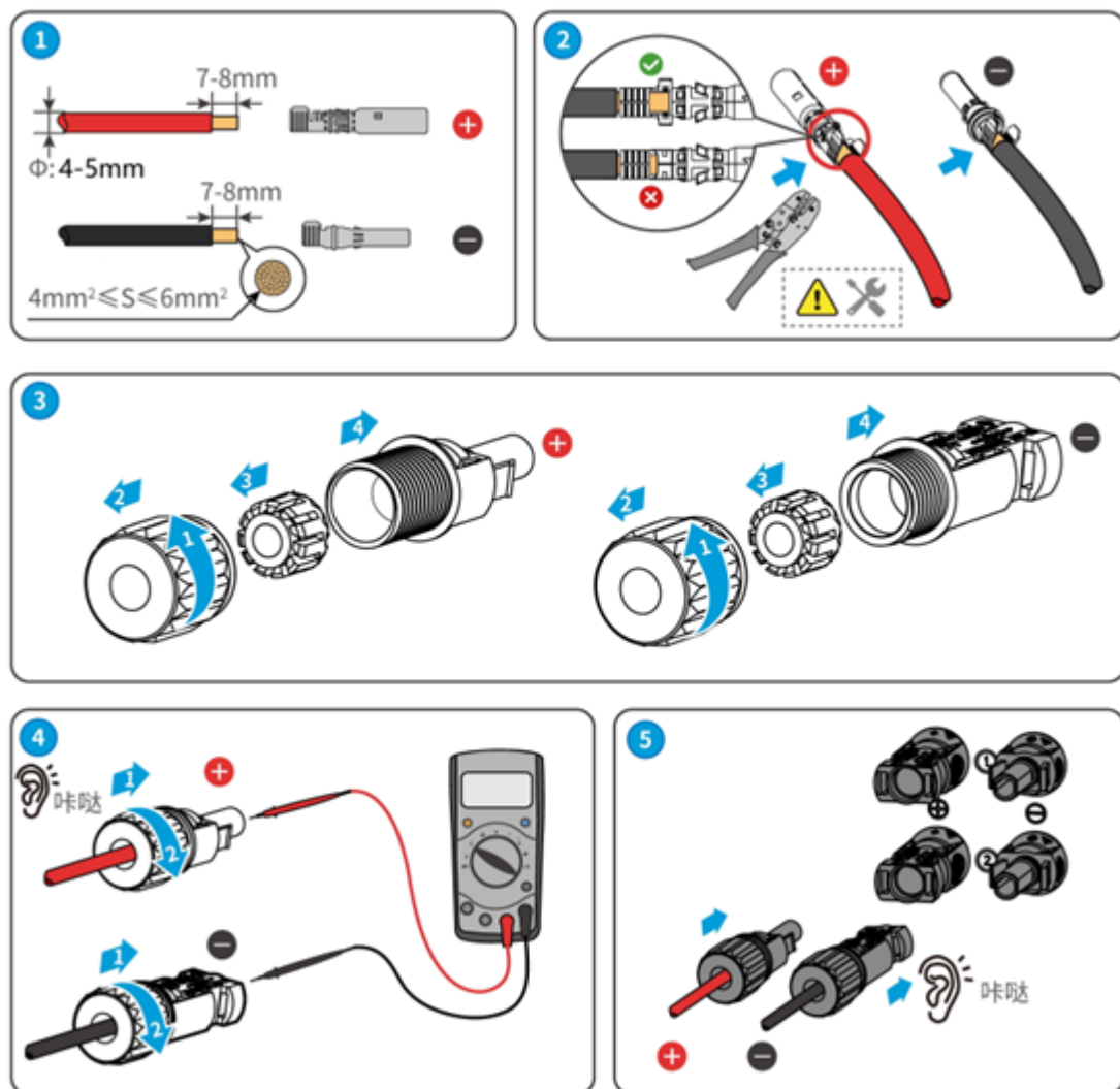
图 6-4 储能机柜PV接线（KYT30kW-108kWh-A为例）
