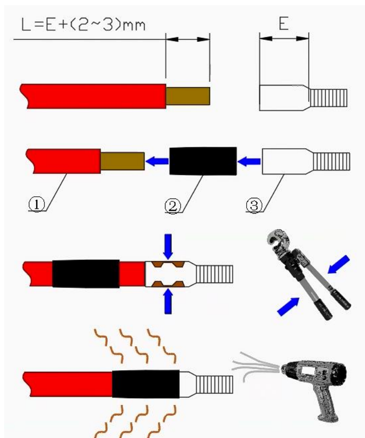
图 6-2 储能机柜交流线压接 ①：线束 ②：热缩管 ③：端子
