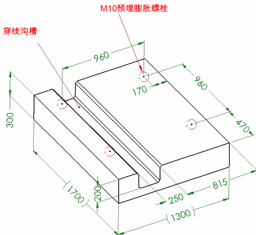
图 5-5 储能机柜设水泥基础形式1尺寸图（单位：mm）
