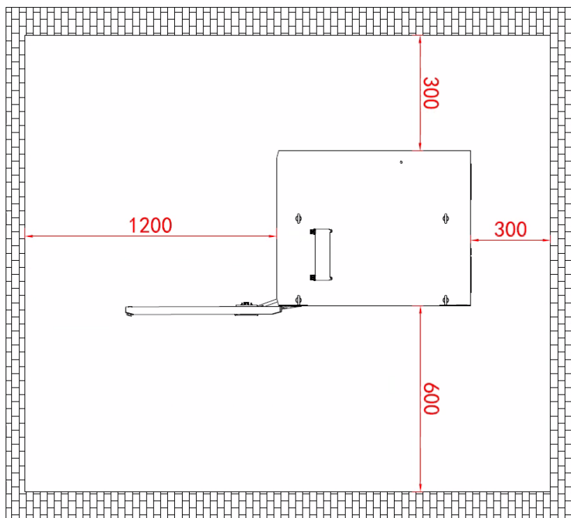
图 5-8 储能机柜周围无遮挡范围尺寸(单位:mm) (KYT30KW-108kWh-A为例)
