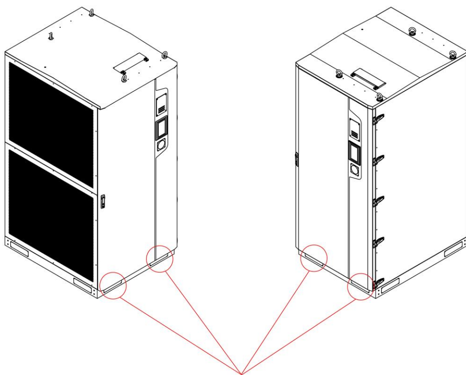
图 5-7 储能机柜固定位置（KYT30KW-108kWh-A为例）
