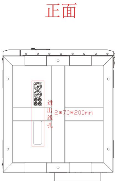
图 3-9 进出线口示意图
